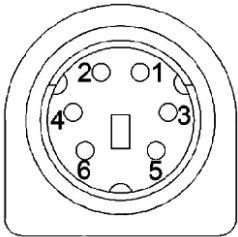
miniDIN (MD6) Steckerdraufsicht miniDIN (MD6) Plug frontview
